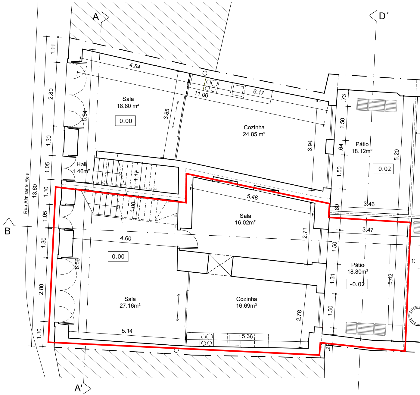
PLANTA R/CHÃO
