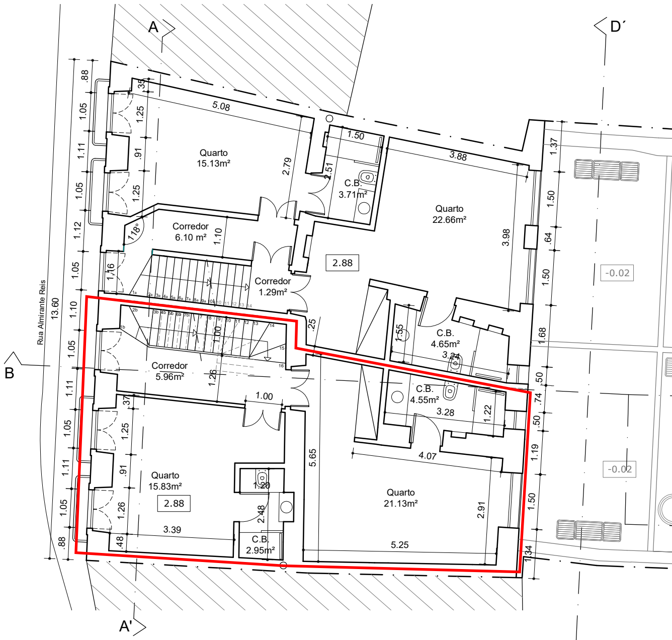
PLANTA 1º ANDAR
