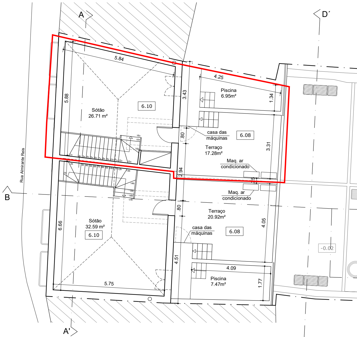
PLANTA SÓTÃO
